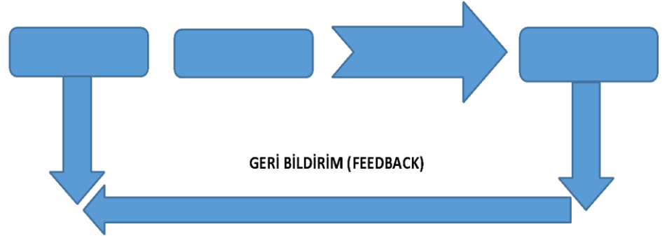
Şekil 12.1. İletişimin Bileşenleri
